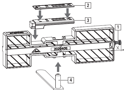
ill.. 8.7: Zarážka a podložky s asymetrickým šroubovým spojem
